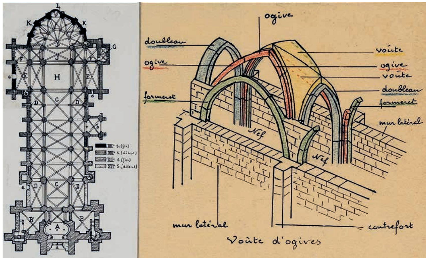
Abb. 3 Der Plan der Kathedrale von Lausanne, der einem dreidimensionalen Schema des Konstruktionsystems eines Kreuzrippengewölbes gegenübergestellt ist, zeugt ebenfalls vom didaktischen Genie des Gelehrten (Tuschezeichnung, Buntstift, Detail ca. 10×16 cm). ACV, PP 100/156. Repro F. Pajor
