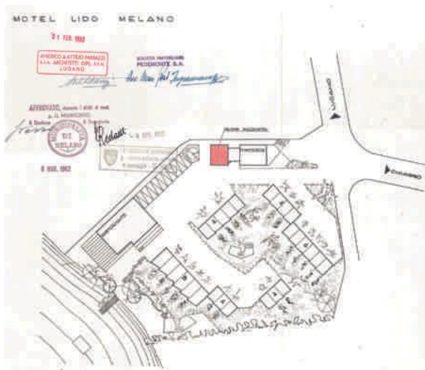
Motel Lido, Melano (1959), progettato da Americo e Attilio Marazzi. Planimetria generale (1962), oggi demolito. Archivio Comunale di Melano
