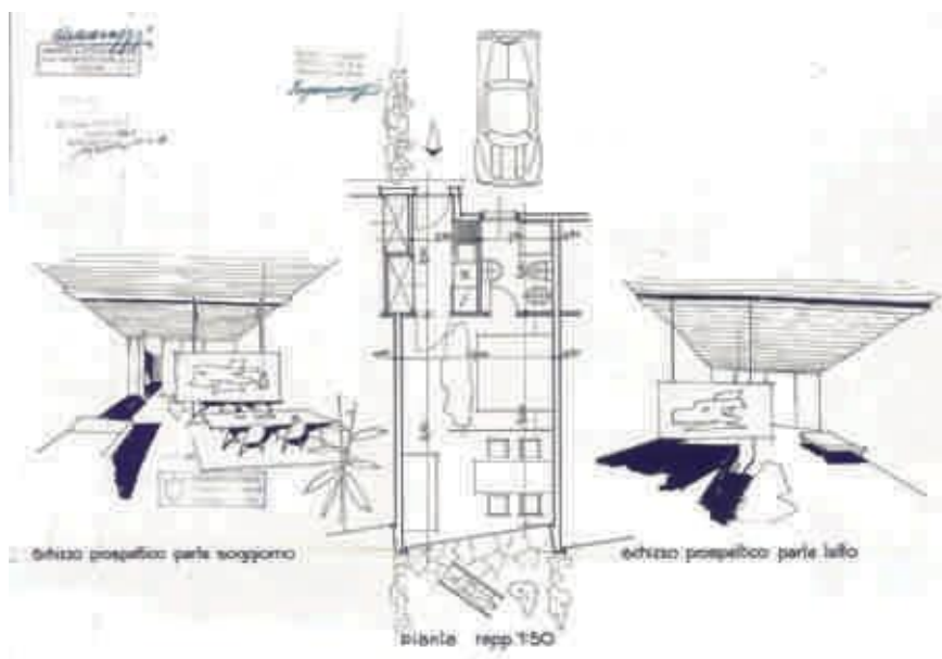
Motel Lido, Melano, «cellula» a tre letti: pianta scala 1:50 e schizzi prospettici. Archivio Comunale di Melano
